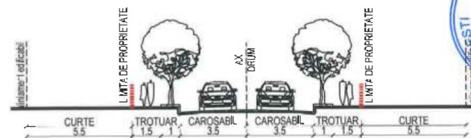
PROFIL STRADAL - STR. AIUD SC. 1:200
