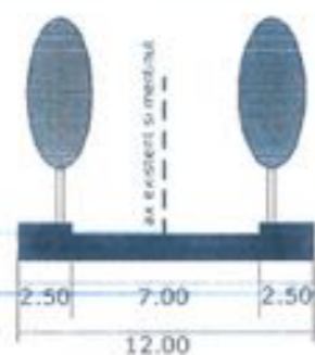
PROFIL EXISTENT STR. CAROL KNAPPE
