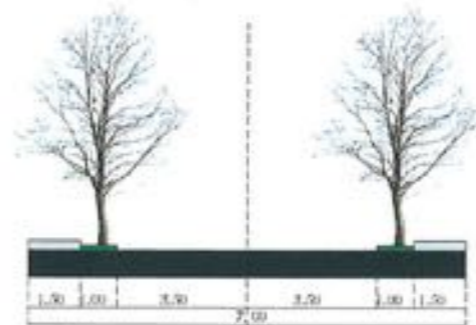
STR. MODESTIEI - PROFIL EXISTENT SI MENTINUT
