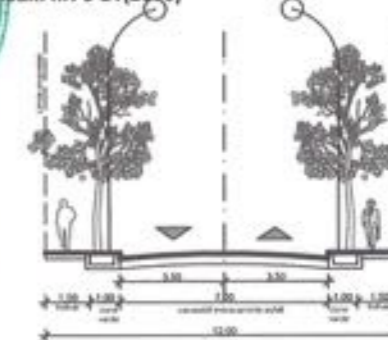
Profil transversal Aleea Teisani - Aprobat prin PUZ Aleea Teisani nr. 3-21(2006)
