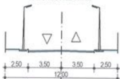
PROFIL TRANSVERSAL SECTIUNEA A-A
