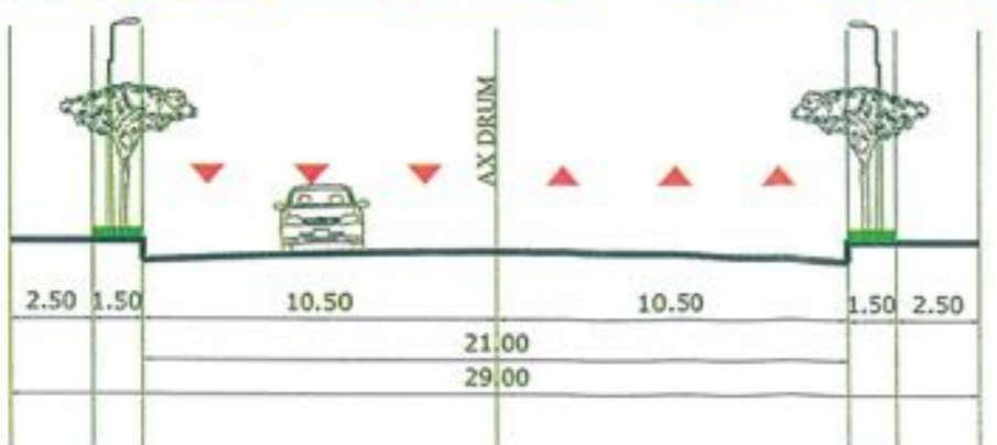
STR. ALEEA PRIVIGHETORILOR Sectiune caracterisita a drumului nou propus conform PUZ APROBAT - Ansamblu Baneasa, sect. I
