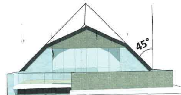
MANSARDA INSCRISA IN PANTA 45° SUPRAFATA MAXIMA 60% DIN AC
