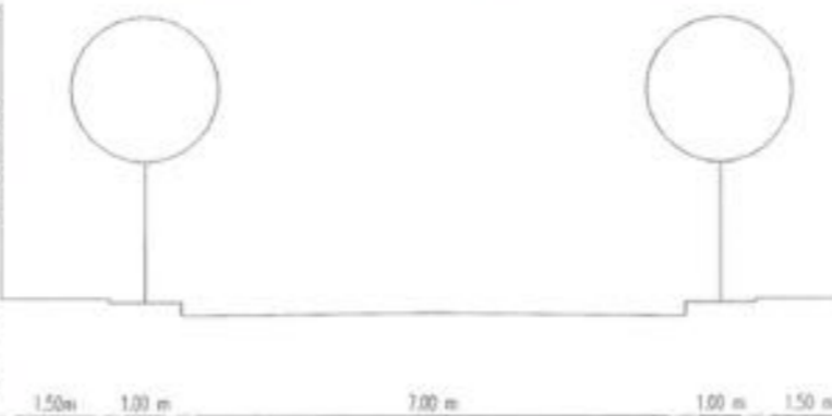
Profil strada Ghita Hagi sc 1:10
