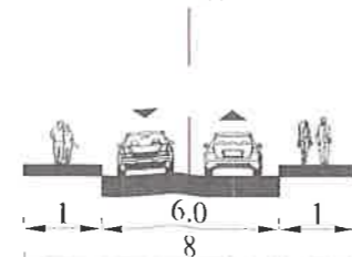
Profil PC 1 - 1 existent și menținut Strada AGAPIA ax menținut
